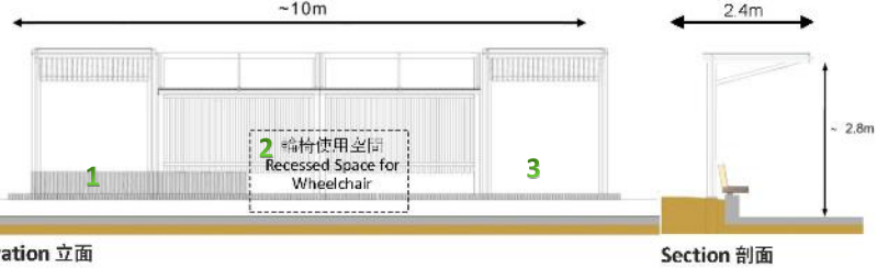
Elevation 立面
