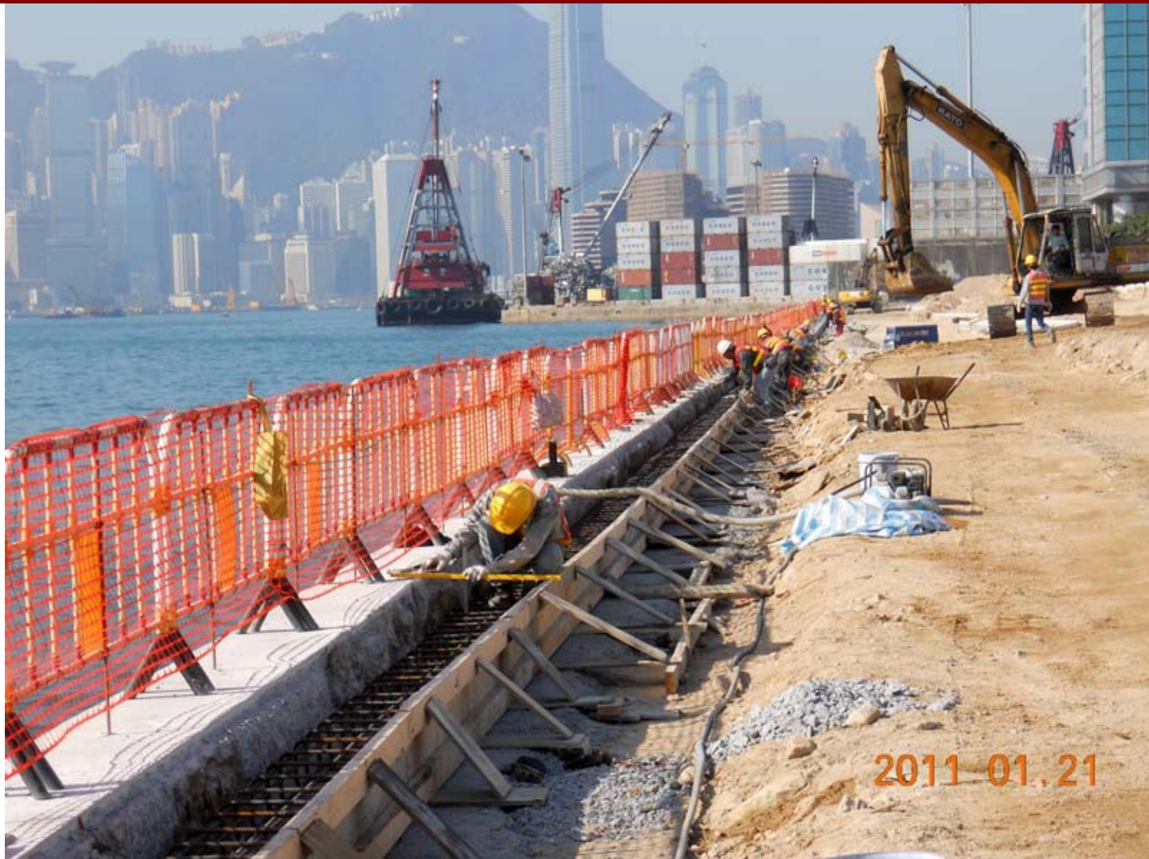
Progress Photo – Railing Footing Construction 進度照片 – 建造欄杆基腳
