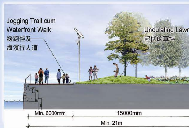
SECTIONAL ELEVATION BB 橫切立面圖 BB
